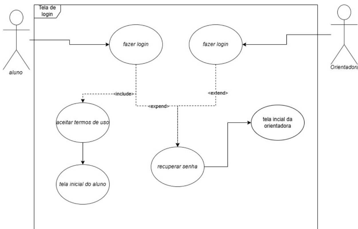
Figura 18 Diagrama de casos de uso 0.0
