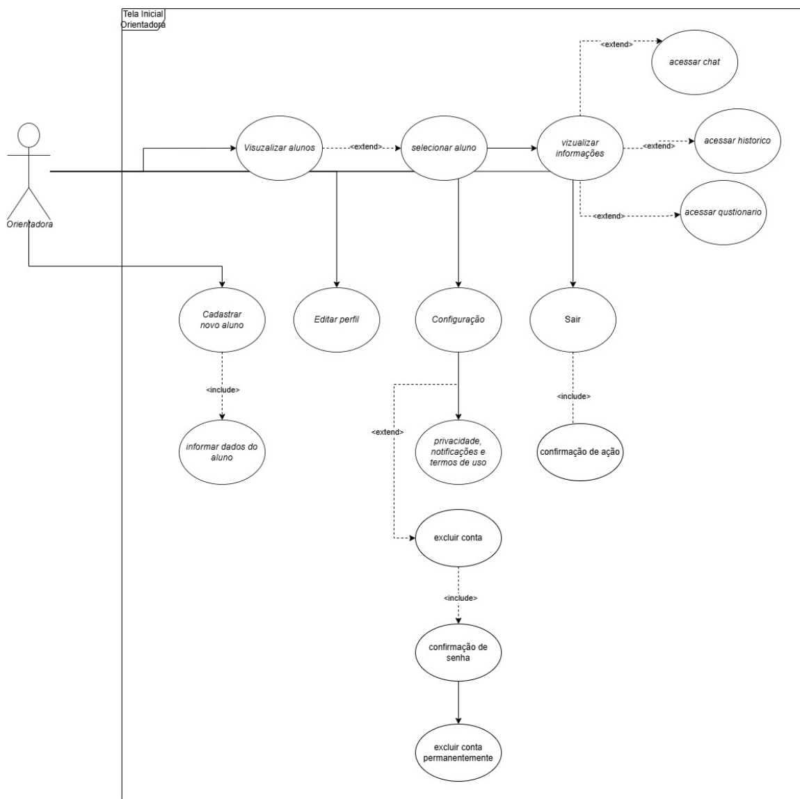
Figura 19 Diagrama de casos de uso 0.1
