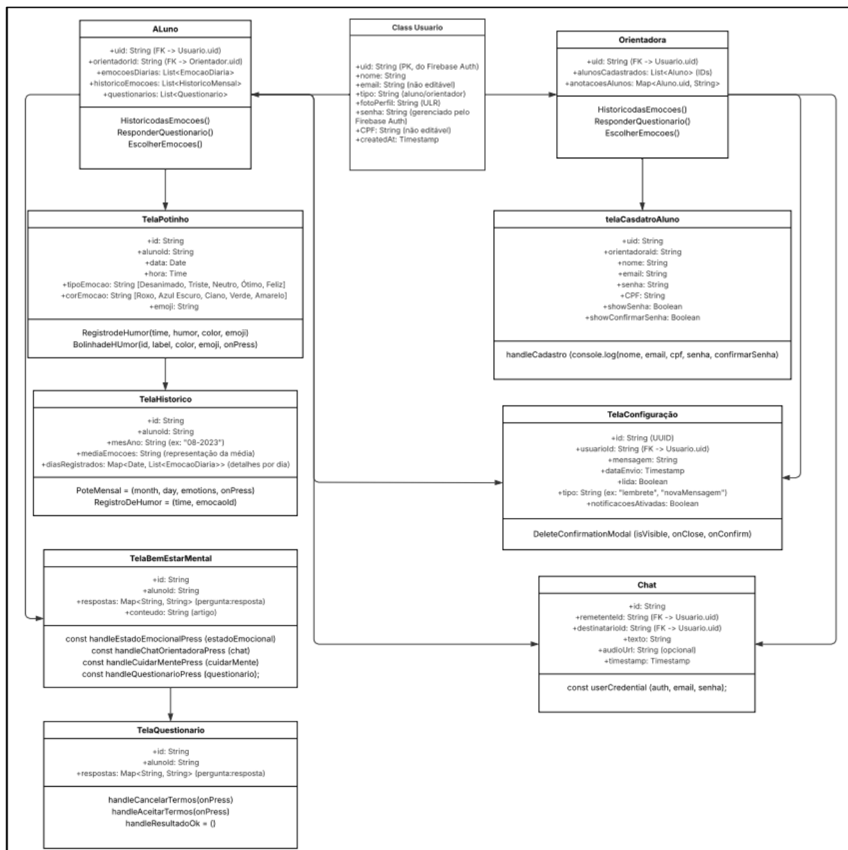
Figura 22 Diagrama de classe
